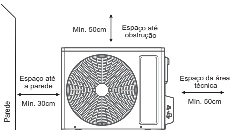
Visualização frontal
