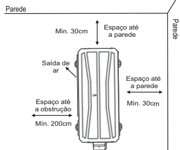
Visualização superior
